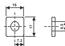
F4 (БОЛТ М6)
