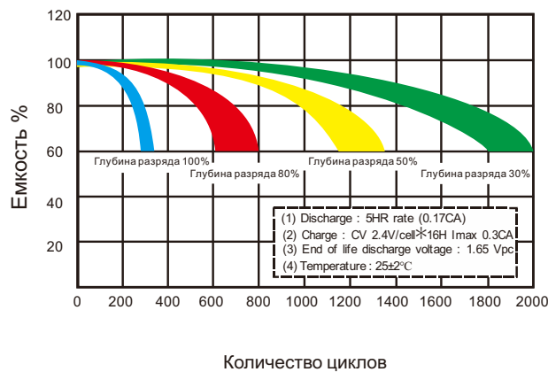
Циклическое использование
