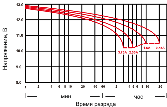
Разрядные характеристики
