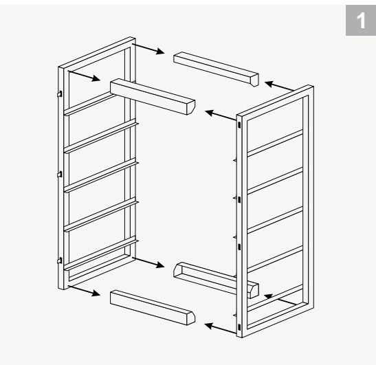
Сборка каркаса
