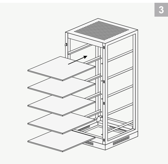
Установка полок
