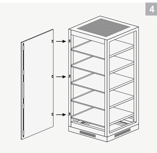
Установка двери
